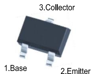
SOT-323
